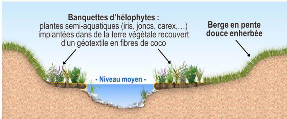
Coupe transversale d'une banquette végétalisée
